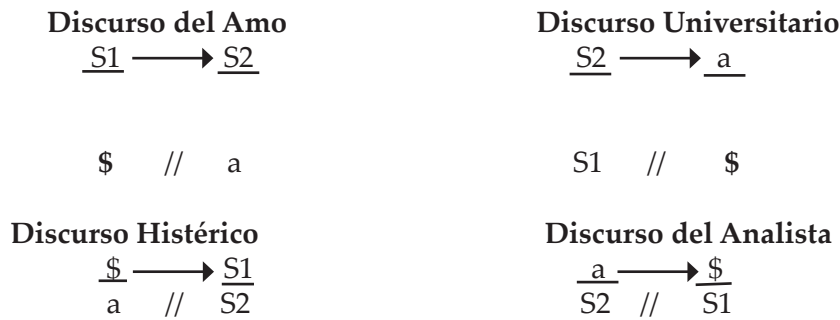
Figura 2: Esquemas del discurso propuestos por Jacques Lacan
